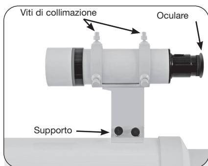
Fig. 14: Gruppo cercatore 8x50
