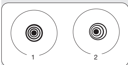
Fig. 32: Collimazione corretta (1) e scorretta (2) osservate durante un test di osservazione di una stella (star test).
