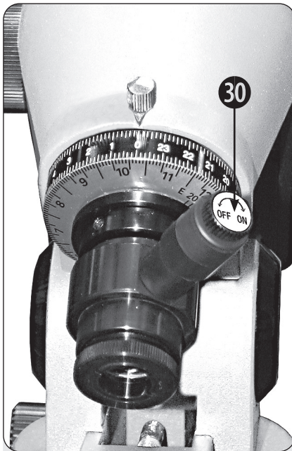
Fig. 37: Vista in dettaglio: cercatore polare con manopola (ON/OFF)
