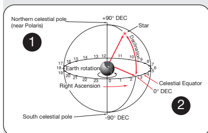
Fig. 33: Sfera celeste
