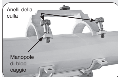
Fig. 8a: Posizionare il tubo ottico negli anelli e stringere leggermente le manopole di bloccaggio degli anelli della culla.
