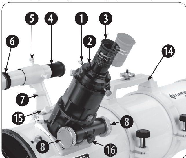
Fig. 1a: le télescope de série Messier inclus un chercheur réticulé type LED à diode (seulement avec les montures EXOS-2); (modèle figuré: tube optique Newton).
