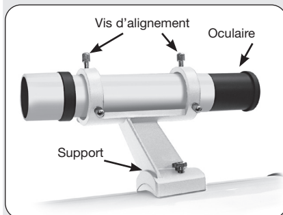
Figure. 14b: 6x30 viseur ensemble de la portée
