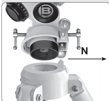
Fig 2d: Fixation de la monture au sommet du trépied
