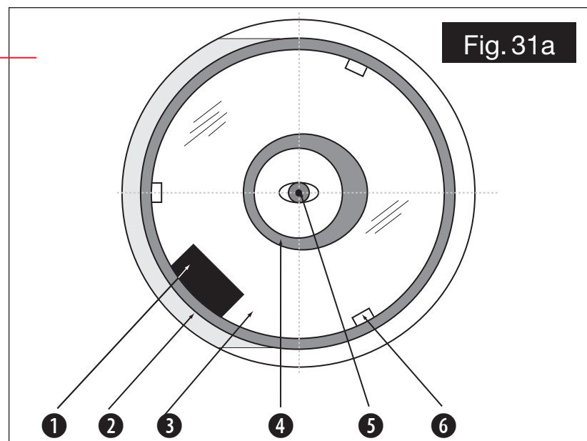
Fig. 31a: un télescope Schmidt-Newton bien collimaté, tel que l'on peut le voir à travers le porte oculaire, sans oculaire.
