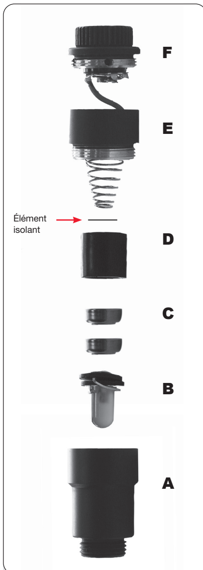
*Fig. 13a: éclaireage du réticule: (A) Compartiment du réticule (B) Diode (C) Piles (D) Porte piles (E) Capot (F) Commutateur „Marche/Arrêt“ (E+F connecté d'un câble)
