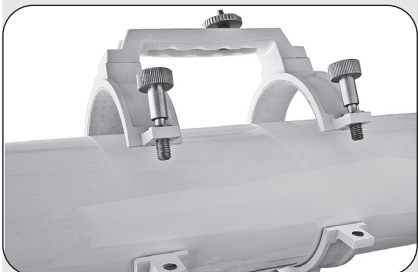
Fig. 2h: Placement du tube optique dans le collier
