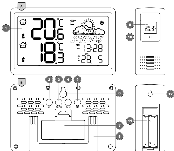
Fig. 1: Aperçu des pièces pour la station de base et le capteur sans fil
