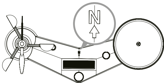
Indicatore del nord sulla parte superiore del sensore 7 in 1.
