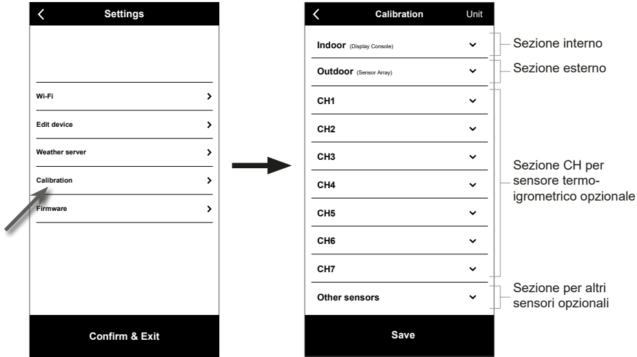
(a) Pagina impostazioni Nella pagina impostazioni, toccare "Calibration".
