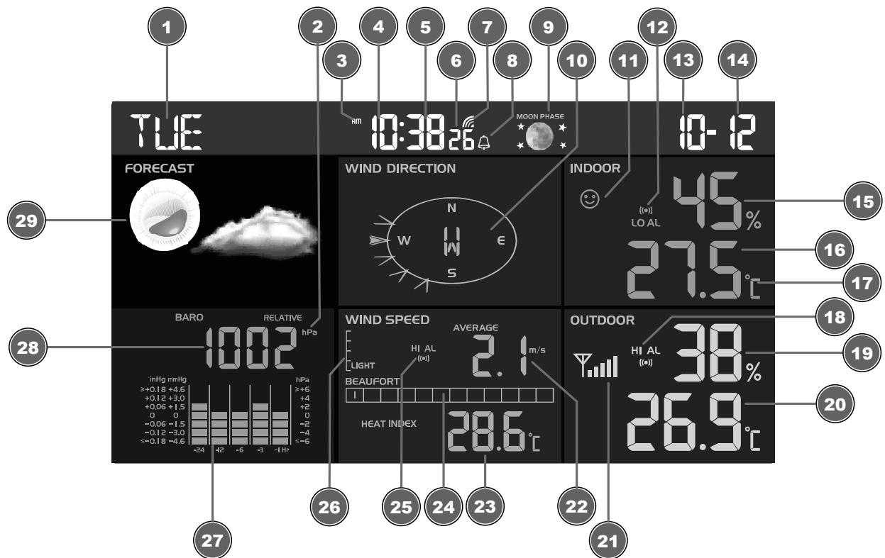
Abb. 2: Display-Anzeigen für die Basisstation
